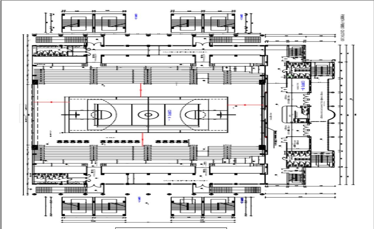
PIANTA LIVELLO
